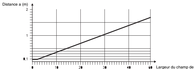
Bild 5.7-3: Distance minimale du barrage immatériel de sécurité mono faisceau par rapport aux surfaces réfléchissantes
