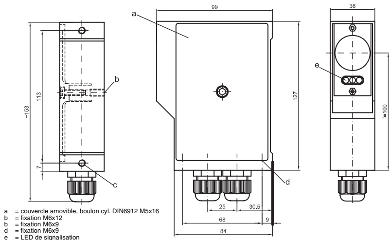
Bild 10.6-1: SLS 78/R avec presse-étoupe PG
