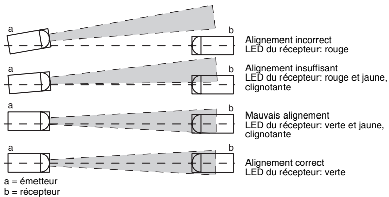
Bild 7.1-1: Contrôle de l'alignement optique
