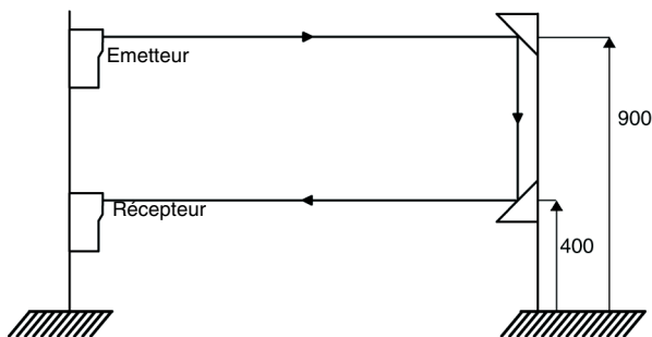
Bild 5.8-1: Ex. 1 pour les utilisations avec miroirs de renvoi, vue latérale
