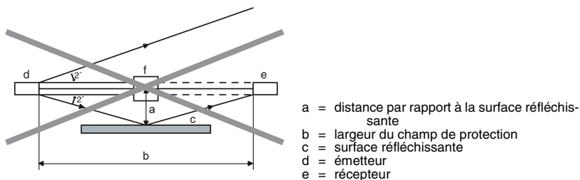
Bild 5.7-1: Mauvaise installation: la déviation entraîne un danger
