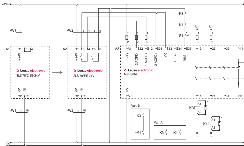
Bild 7.0-1: Ex.: SLS 78/R avec MSI-SR4
