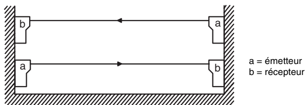
Bild 5.5-1: Agencement multiaxe
