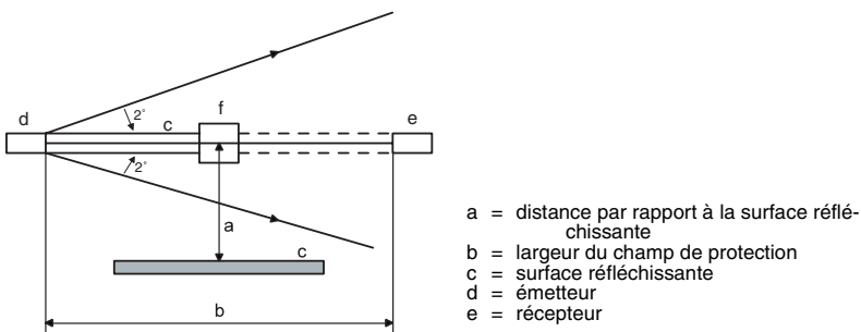
Bild 5.7-2: Installation correcte: la déviation n'entraîne aucun danger
