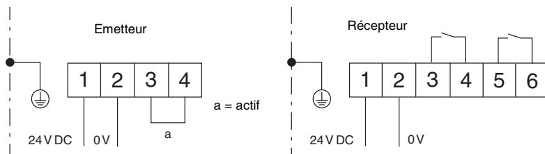
Bild 6.2-1: Connexion de la version à bornes
