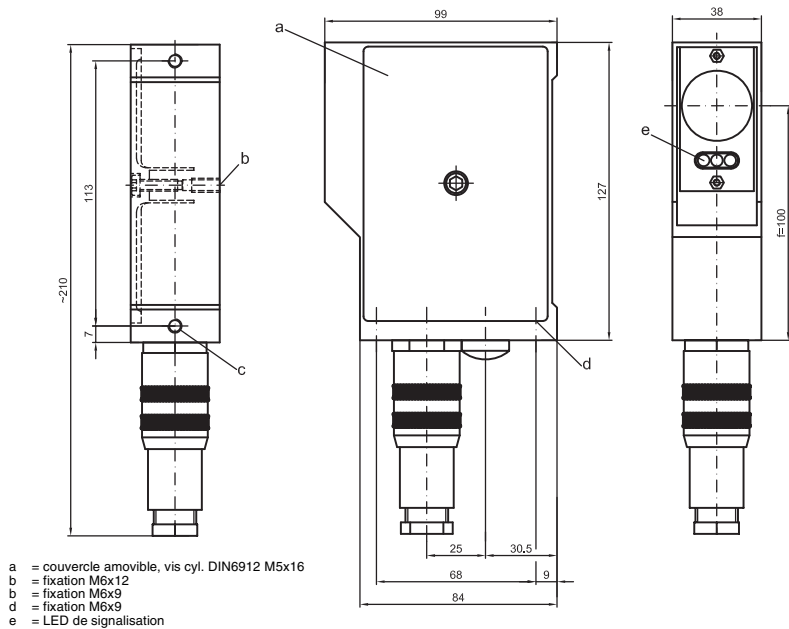
Bild 10.6-2: SLS 78/R avec connecteur selon la norme DIN 43651
