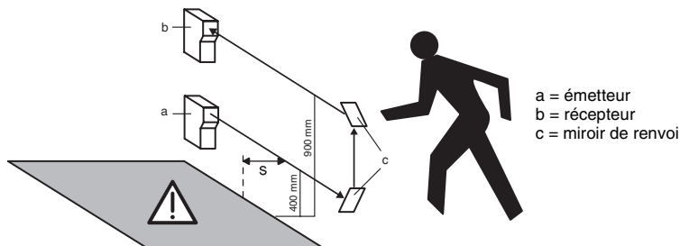
Bild 5.2-1: Distances de sécurité
