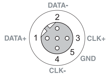
M12-Buchse (B-codiert)
